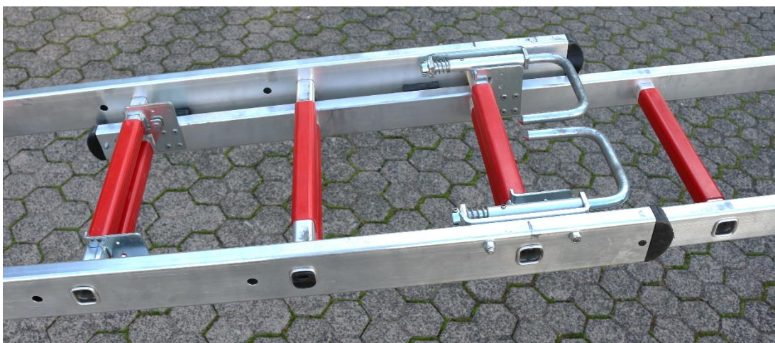
Abbildung 35: Arretiertes Aufsteckteil
